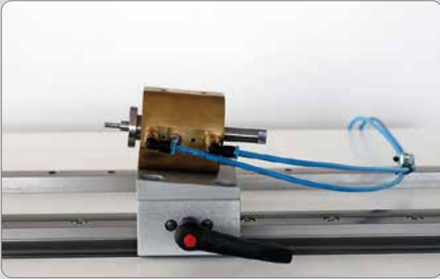
PMB Luftlager für hochgenaue Wellenwuchtung
